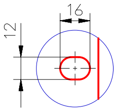
Detalle A (x4) Escala 1:2
